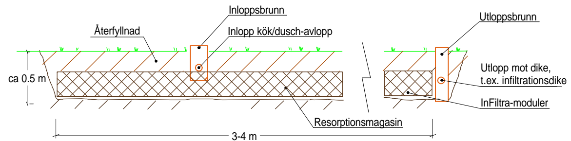
LÄNGDSEKTION
