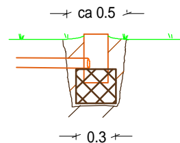
TVÄRSEKTION
